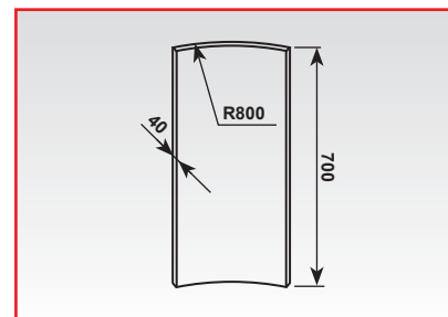
Radius 800 síla 40 mm 1/8 oblouku
