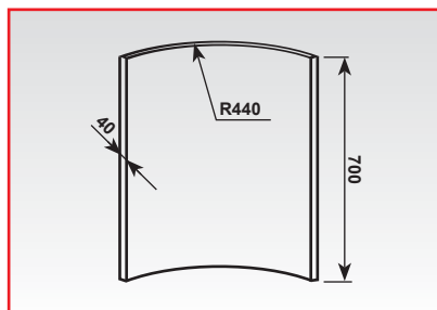
Radius 440 síla 40 mm 1/4 oblouku
