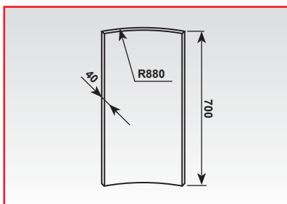
Radius 880 síla 40 mm 1/8 oblouku
