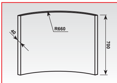
Radius 660 síla 40 mm 1/4 oblouku
