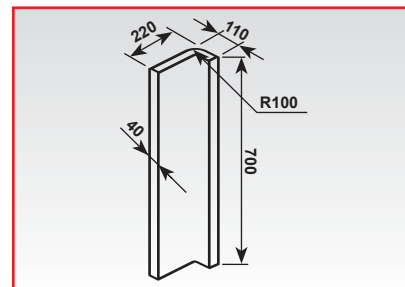
Roh díl 90° R 100/40 mm výška 700 mm 220/110mm
