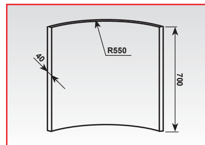
Radius 550 síla 40 mm 1/4 oblouku
