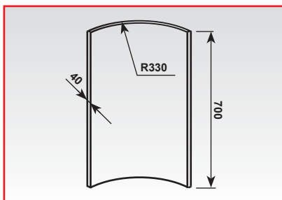
Radius 330 síla 40 mm 1/4 oblouku
